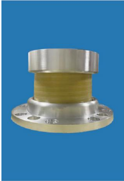
110kV
